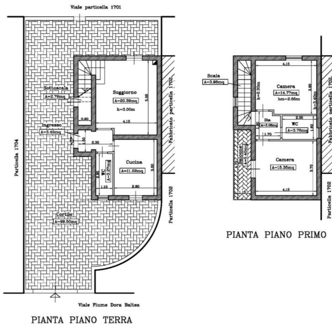
Immagine n. 2 – Pianta
