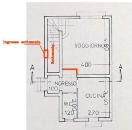
PIANTA PIANO TERRA Come da P.d.C. n. 129/08
