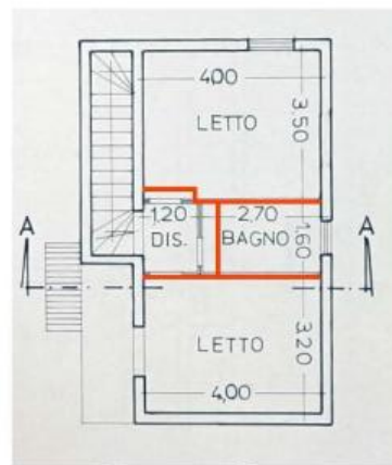
PIANTA PIANO PRIMO Come da P.d.C. n. 129/08
