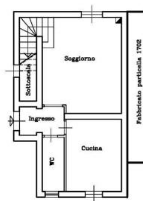
PIANTA PIANO TERRA Come da rilievo
